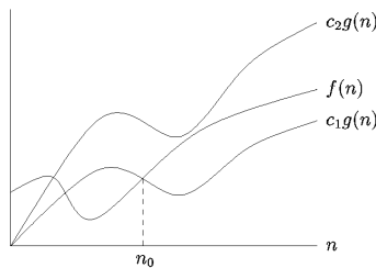
Σχήμα 2.5: f = \Theta(g)
