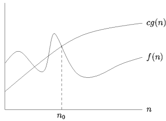
Σχήμα 2.3: f = O(g)
