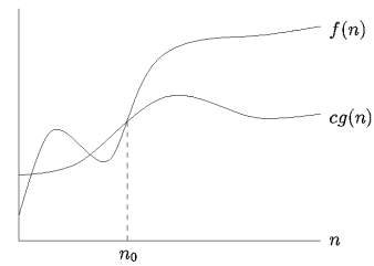
Σχήμα 2.4: f = \Omega(g)
